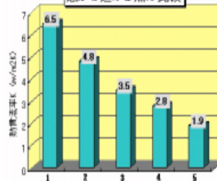
窓から逃げる熱の比較
